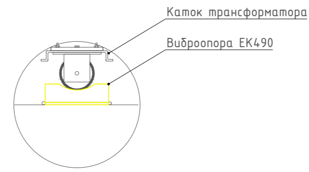
Узел установки трансформатора на виброопоре
